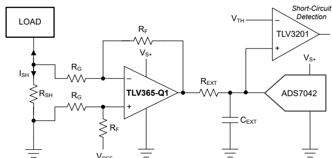
TLVx365-Q1 用于电流检测
