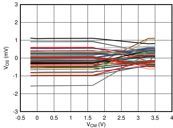
图 5-3. V_{OS} vs V_{CM} @ V_{CC} = 3.3\text{V} - 50 Devices
