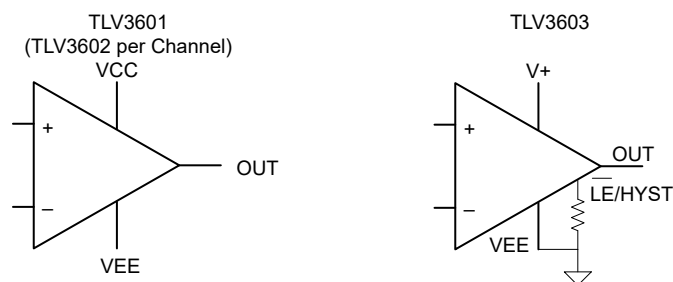
功能方框图
