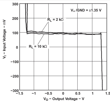
图 5-12. 输入电压与输出电压间的关系
