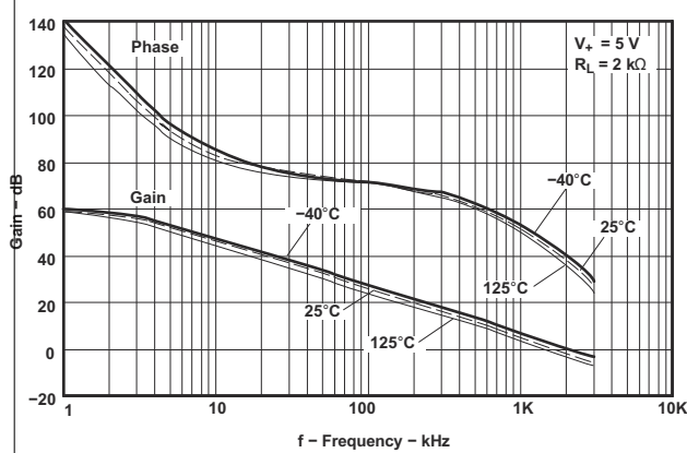
图 5-21. 频率响应与 温度间的关系
