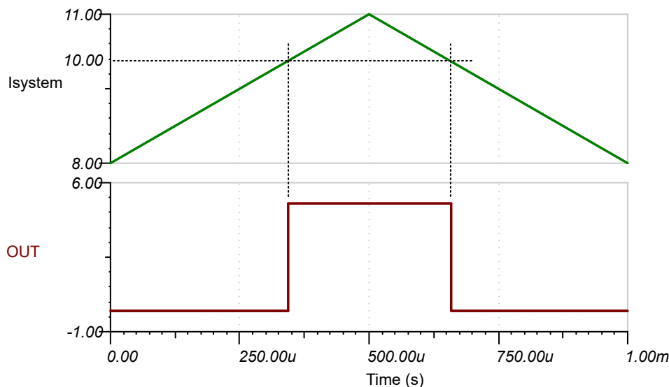
图 7-8. 过流结果
