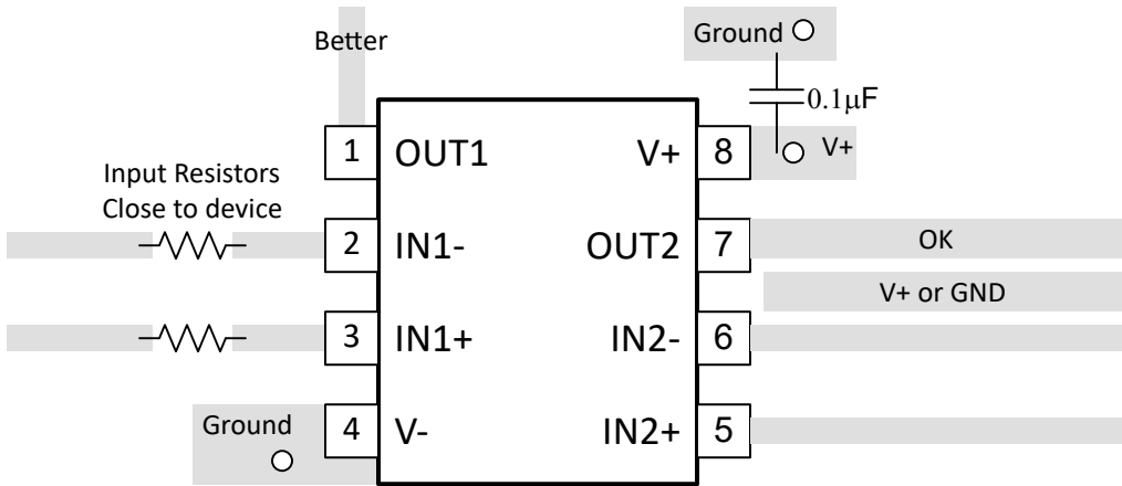
图 7-9. 双通道布局示例
