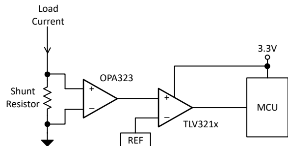
低侧电流检测
