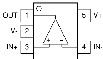
DCK、DBV 封装 SC70 , SOT-23-5 顶视图 ( 西北引脚排列 )
