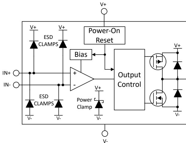
图 6-1. TLV321x 推挽方框图
