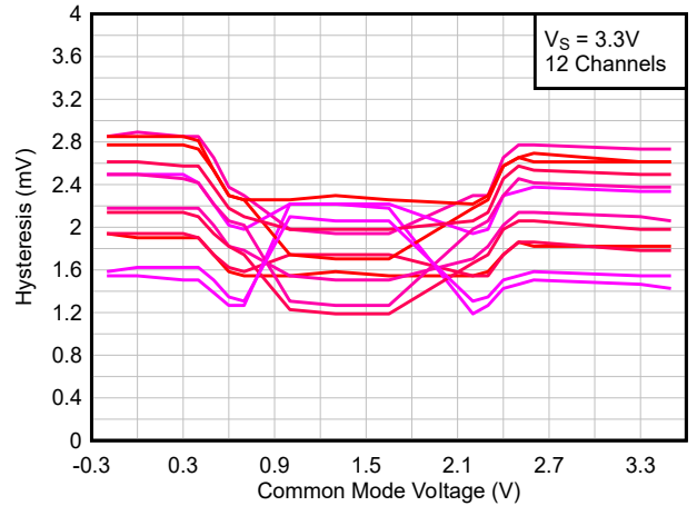
图 5-10. 迟滞与 共模电压间的关系, 3.3V
