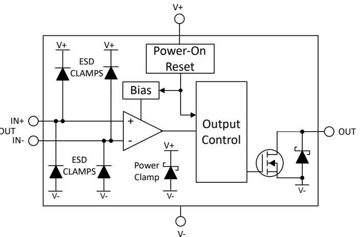
图 6-2. TLV322x 开漏方框图
