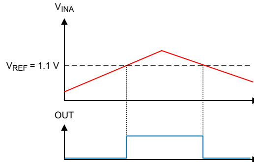
图 7-8. 过流结果
