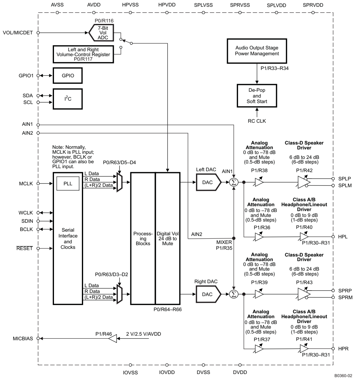
图 1-1. 功能方框图
