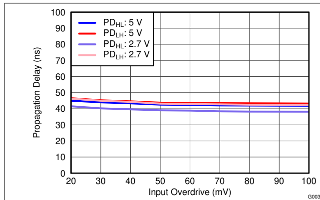
图 6-19. 传播延迟与输入过驱间的关系
