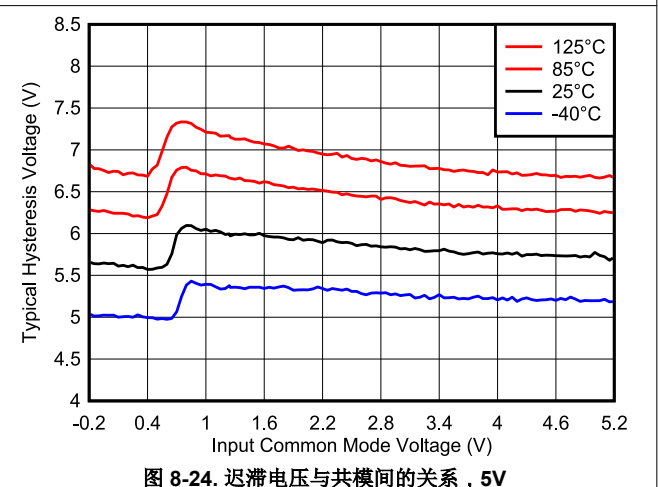
图 8-24. 迟滞电压与共模间的关系, 5\text{V}
