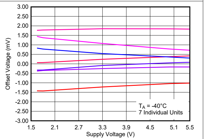
图 8-34. 失调电压与电源电压间的关系, -40°C
