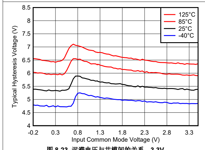
图 8-23. 迟滞电压与共模间的关系, 3.3\text{V}
