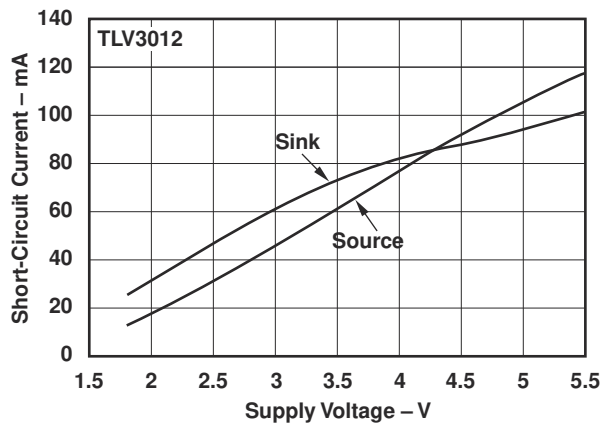
图 7-19. 短路电流与电源电压间的关系
