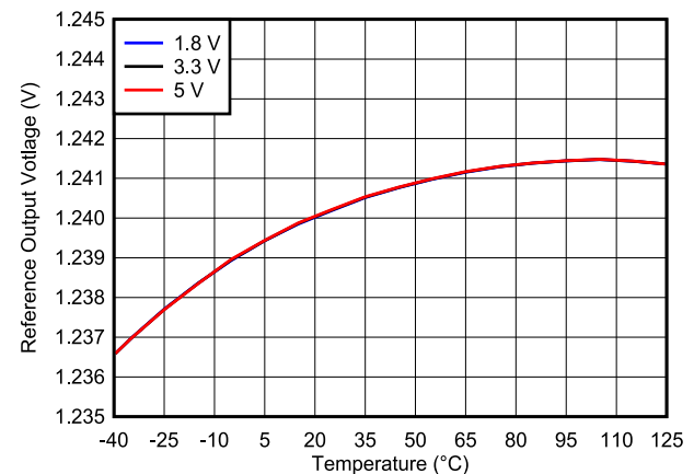
TLV3012B-Q1 基准电压与温度间的关系
