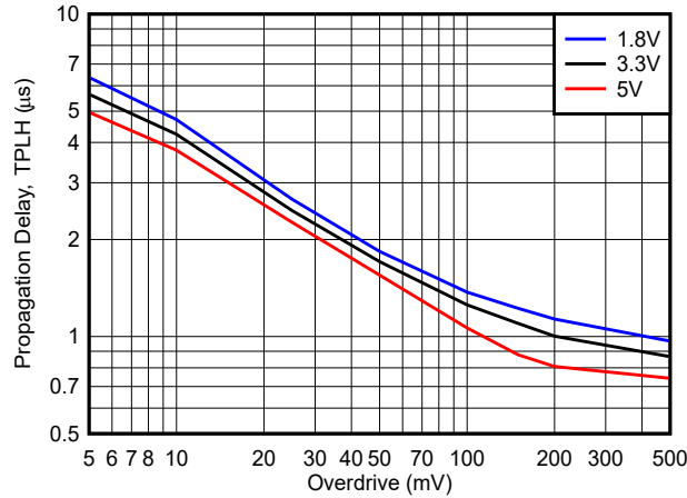
图 6-13. 从低电平到高电平传播延迟时间与过驱间的关系
