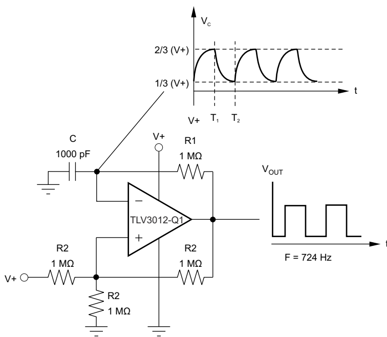
图 8-6. TLV3012-Q1 配置为张弛振荡器
