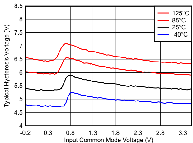
图 6-23. 迟滞电压与共模间的关系, 3.3V
