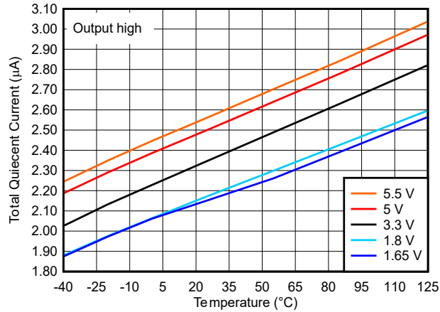
图 6-7. 电源电流与温度间的关系
