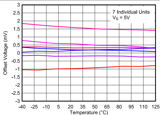
图 6-28. 失调电压与温度间的关系, 5V
