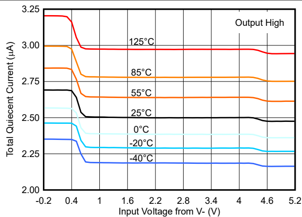
图 6-11. 电源电流与共模间的关系 - 5V
