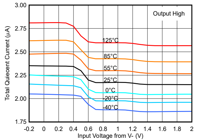
图 6-10. 电源电流与共模间的关系 - 1.8V
