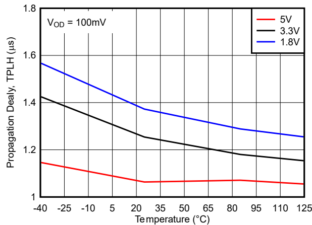
图 6-15. 从低电平到高电平传播延迟时间与温度间的关系
