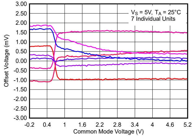
图 6-31. 失调电压与共模电压间的关系, 5V
