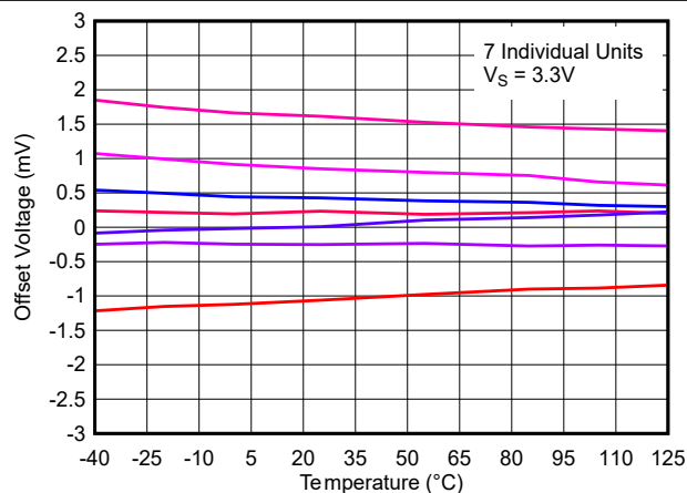
图 6-27. 失调电压与温度间的关系, 3.3V
