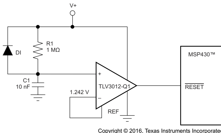
图 8-5. TLV3012-Q1 配置为 MSP430™ 微控制器的上电复位电路
