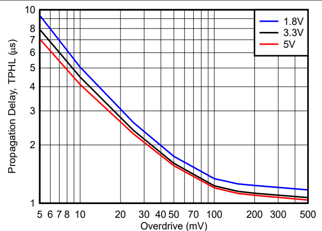
图 6-12. 从高电平到低电平传播延迟时间与过驱间的关系
