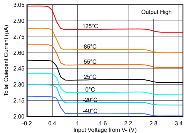
图 6-9. 电源电流与共模间的关系 - 3.3V
