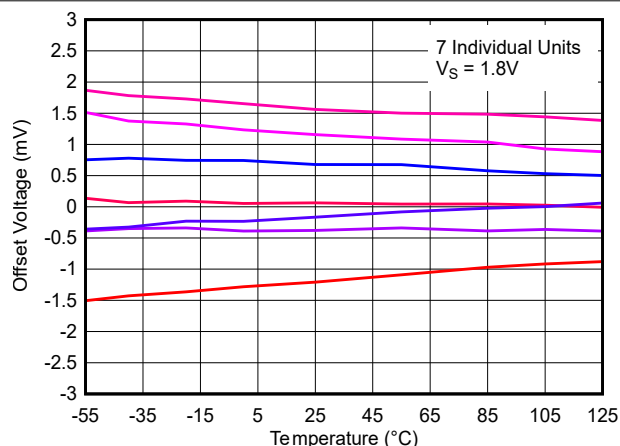
图 6-26. 失调电压与温度间的关系, 1.8V
