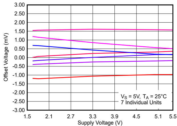
图 6-33. 失调电压与电源电压间的关系, 25°C
