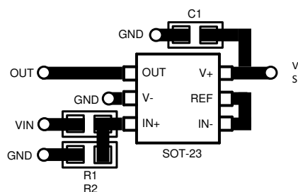
图 8-7. 布局示例
