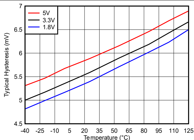
图 6-25. 迟滞电压与电源电压间的关系
