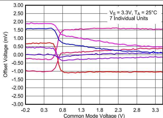
图 6-30. 失调电压与共模电压间的关系, 3.3V
