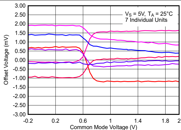
图 6-29. 失调电压与共模电压间的关系, 1.8V
