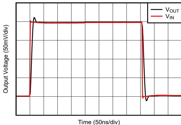
图 6-17. 小信号阶跃响应
