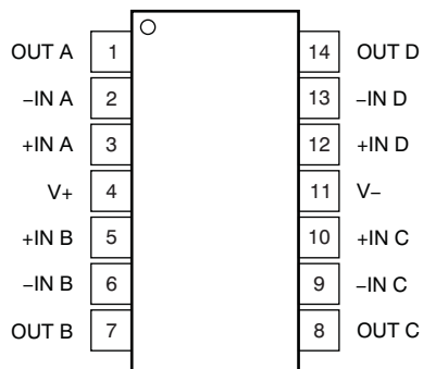
PW 封装 : TLV4333 14 引脚 TSSOP 俯视图
