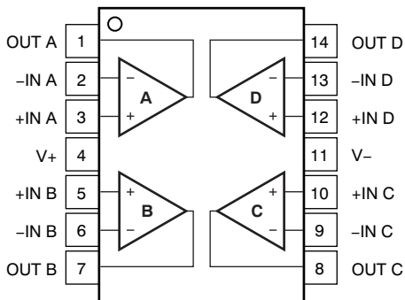
D 封装 : TLV4333 14 引脚 SOIC 俯视图
