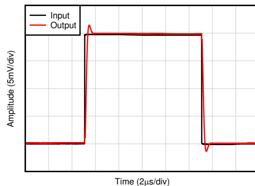
图 5-40. 电压输出器微小信号脉冲响应 (旧裸片) (17)
