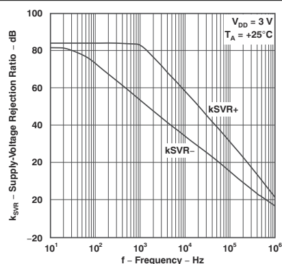
图 5-30. 电源电压抑制比与频率之间的关系 (旧裸片) (12)
