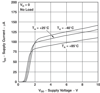
图 5-35. 电源电流与电源电压间的关系 (旧裸片) (14)
