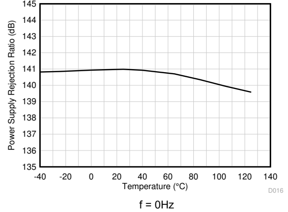
图 5-34. PSRR 与温度间的关系 (dB) (新裸片)
