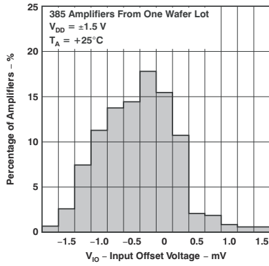
图 5-1. TLV2221 输入失调电压分布 (旧裸片)
