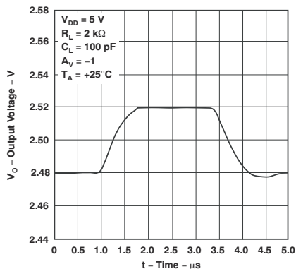
图 5-39. 反相小信号脉冲响应 (旧裸片) (17)
