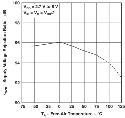
图 5-33. 电源电压抑制比与自然通风温度间的关系 (旧裸片)
