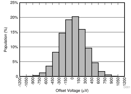
图 5-2. TLV2221 输入失调电压分布 (新裸片)
