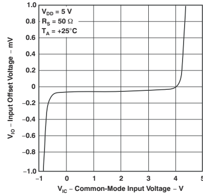
图 5-4. 输入失调电压与共模输入电压间的关系 (旧裸片) (1)
