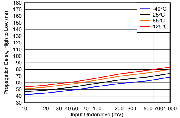
图 5-28. 传播延迟 (高电平到低电平) 与输入欠驱间的关系, 12V
