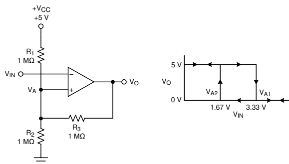
图 7-3. 采用反相配置、具有迟滞功能的 TLV183x-Q1
