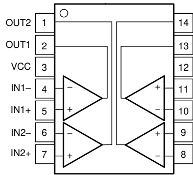
DYY 封装 14 引脚 SOT-23 顶视图
