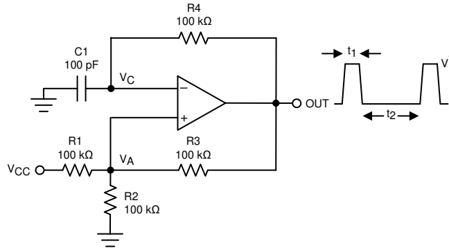
图 7-9. 方波振荡器
