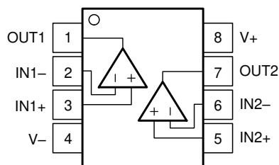
DDF 封装 8 引脚 SOT23-8 顶视图
