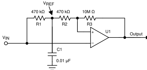
图 7-18. 脉冲切片器
