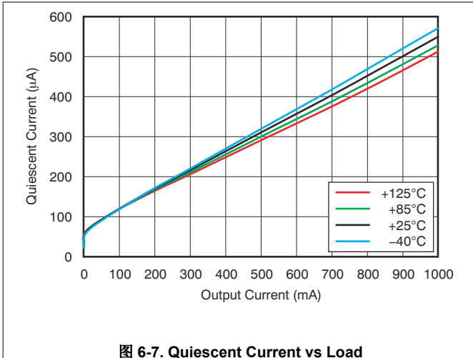
图 6-7. Quiescent Current vs Load
