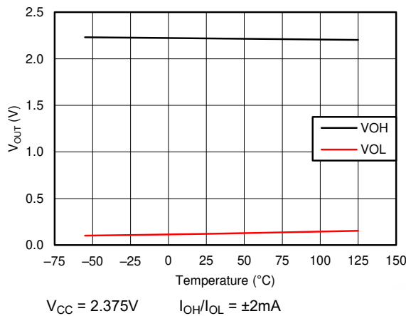
图 7-2. V_{OH}/V_{OL} vs Temperature
