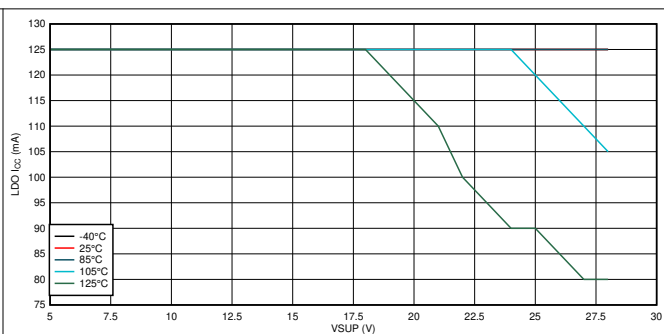
图 7-2. I_{CC} vs V_{SUP} vs Temperature
