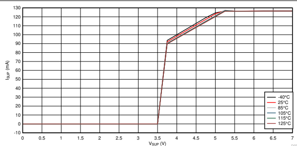
图 10-5. I_{SUP} vs V_{SUP} vs Temperature
