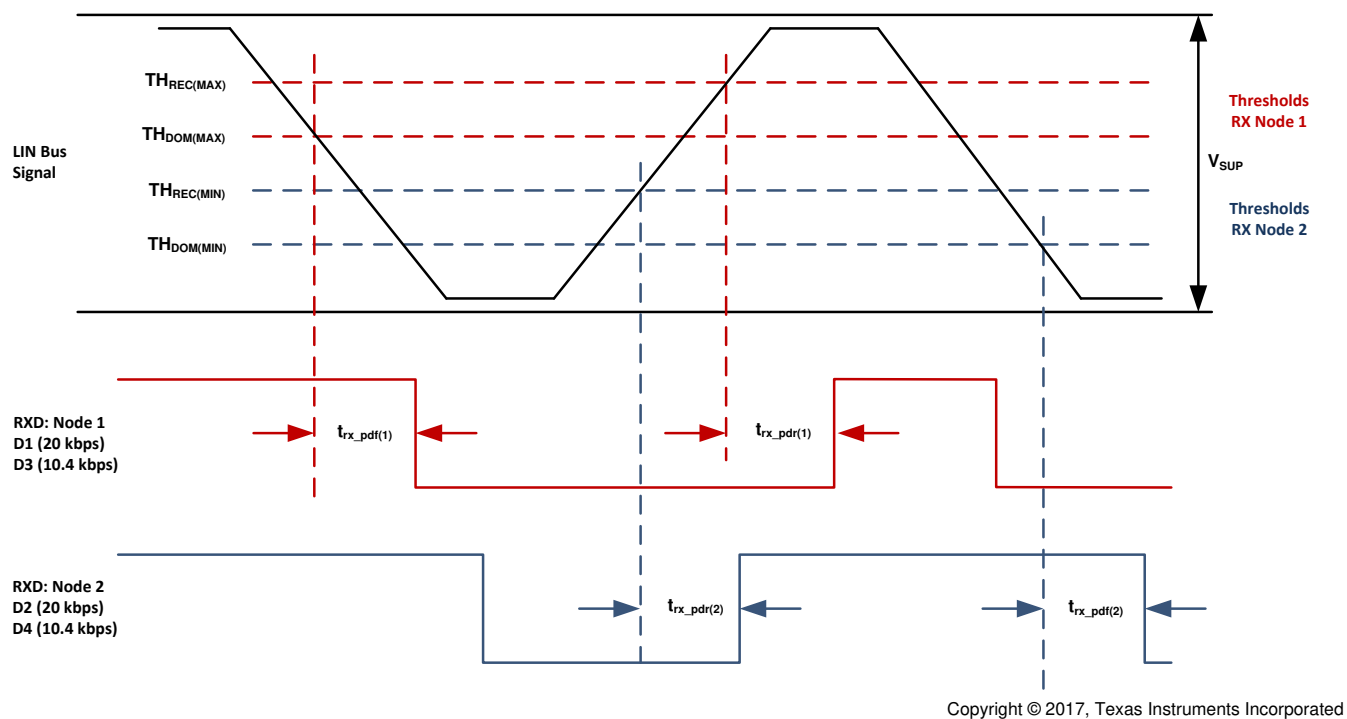
图 8-14. Propagation Delay
