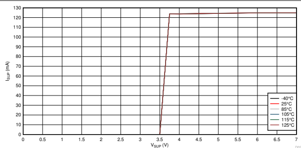
图 10-2. I_{SUP} vs V_{SUP} vs Temperature
