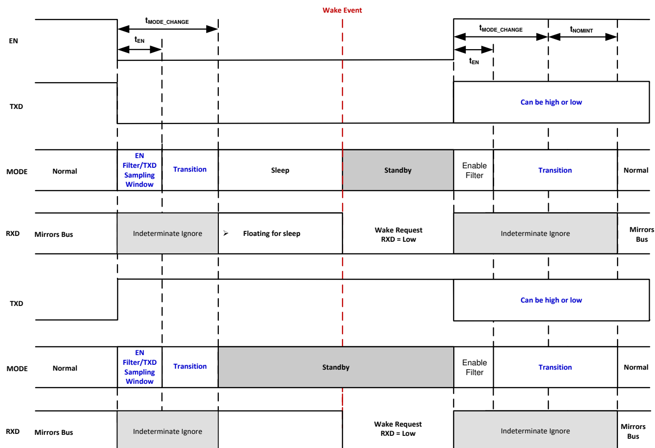
图 8-15. Mode Transitions
