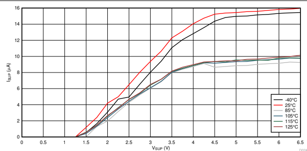
图 10-8. I_{SUP} vs V_{SUP} vs Temperature Ramp-down
