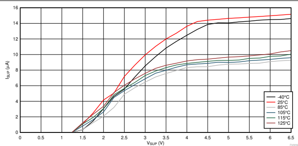
图 10-9. I_{SUP} vs V_{SUP} vs Temperature Ramp-down
