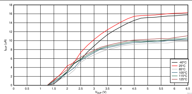
图 10-10. I_{SUP} vs V_{SUP} vs Temperature Ramp-down
