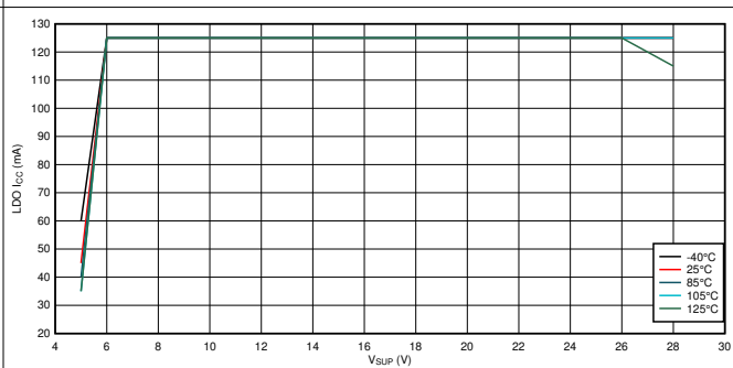
图 7-4. I_{CC} vs V_{SUP} vs Temperature
