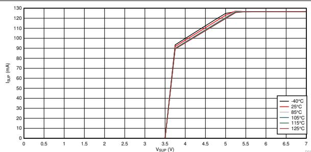
图 10-4. I_{SUP} vs V_{SUP} vs Temperature
