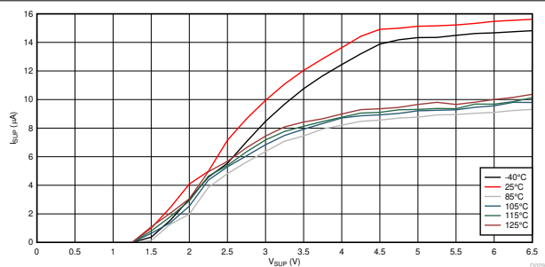
图 10-11. I_{SUP} vs V_{SUP} vs Temperature Ramp-down
