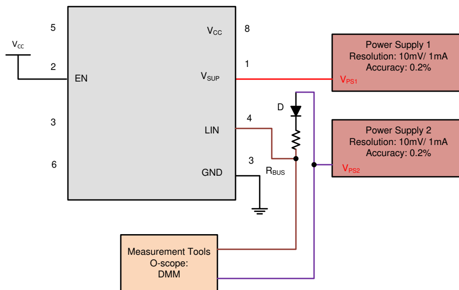
图 8-5. V_{SUP\_NON\_OP} Test Circuit
