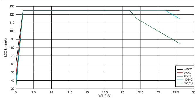
图 7-3. I_{CC} vs V_{SUP} vs Temperature
