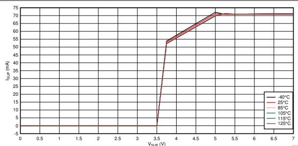
图 10-3. I_{SUP} vs V_{SUP} vs Temperature
