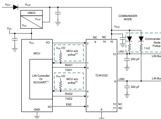
简化版原理图，指挥官模式
