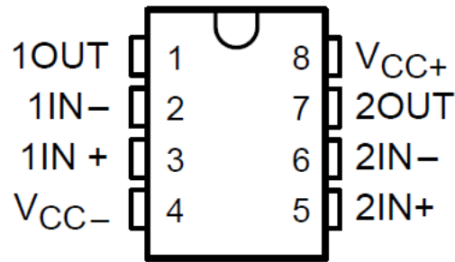
图 5-2. TLE2082D 或 P 封装 ( 顶视图 )
