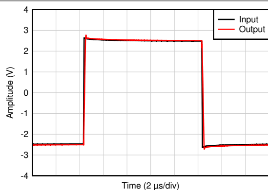
图 6-13. 小信号脉冲响应
