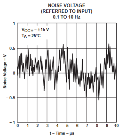
图 5-11. 噪声电压
