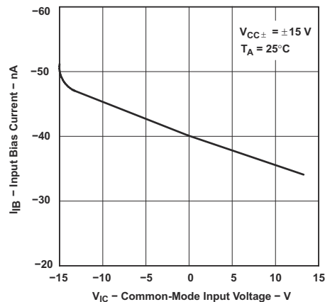
图 6-4. TLE2021 输入偏置电流与共模输入电压间的关系
