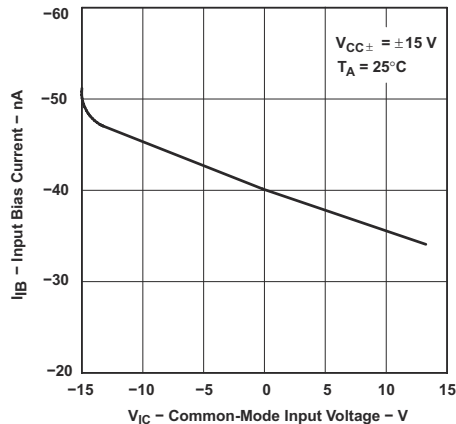
图 5-4. TLE2021xM 输入偏置电流与共模输入电压间的关系
