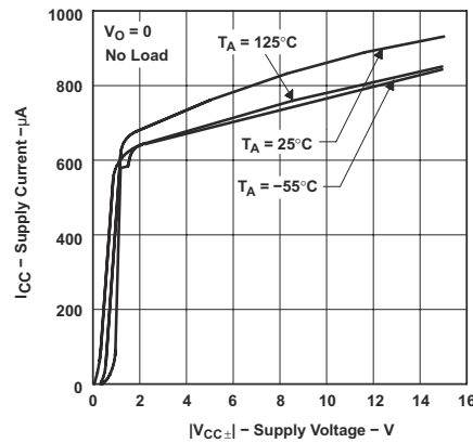
图 5-34. TLE201xM 电源电流与电源电压间的关系
