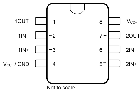
图 4-2. TLE2022xM : JG 封装, 8 引脚 CDIP ( 俯视图 )
