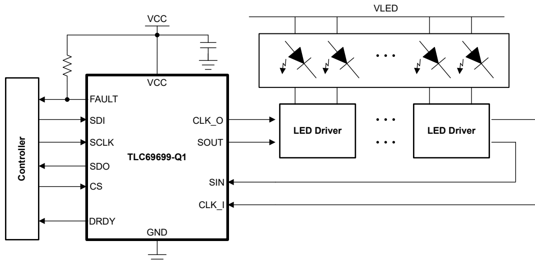
图 3-1. 典型应用图
