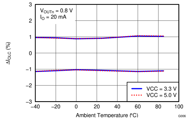
图 5-9. \Delta I_{OLC} 与环境温度间的关系
