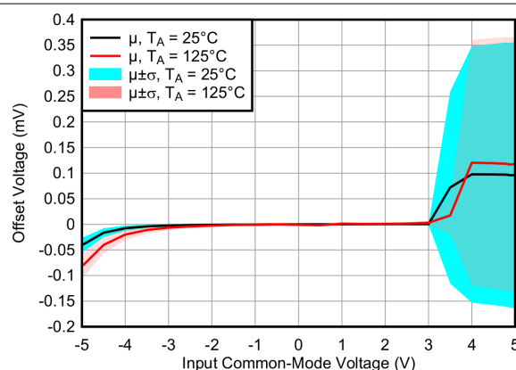
图 7-4. 失调电压与输入共模电压间的关系
