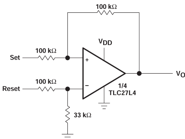
图 7-10. 设置/复位触发器, V_{DD} = 5\text{V} 至 16\text{V}
