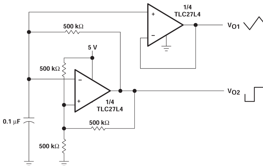
图 7-9. 多谐振荡器
