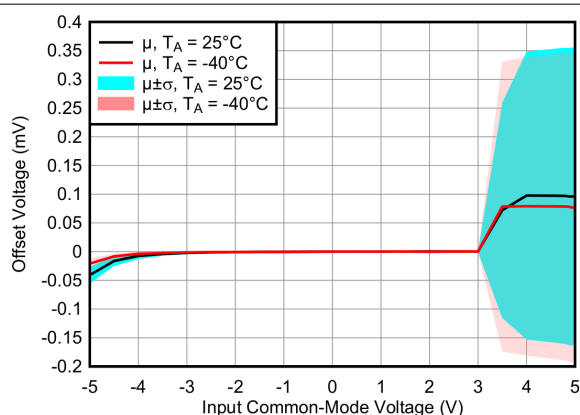
图 7-3. 失调电压与输入共模电压间的关系
