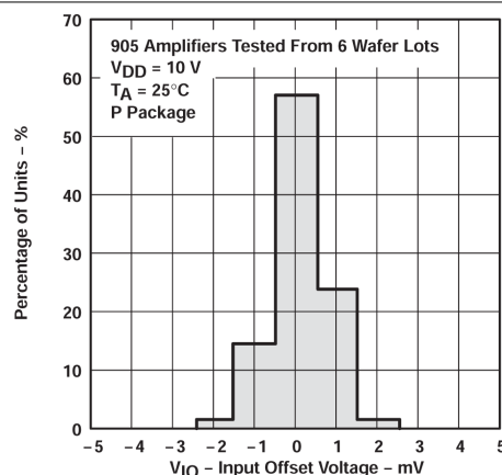
图 5-2. TLC27L2 输入失调电压的分布
