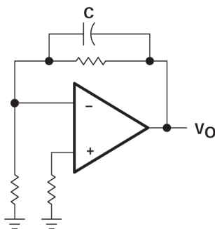
图 7-6. 对输入电容进行补偿
