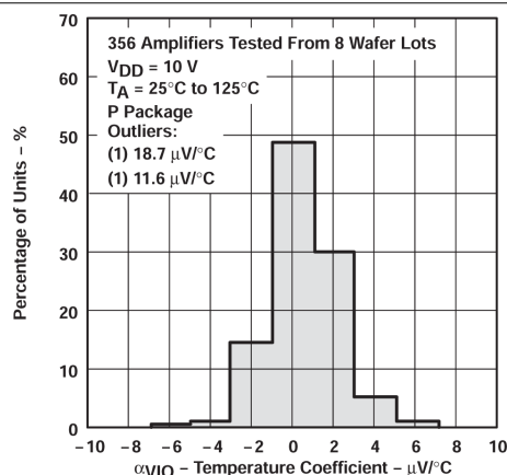
图 5-4. TLC27L2 与 TLC27L7 输入偏移电压温度系数的分布
