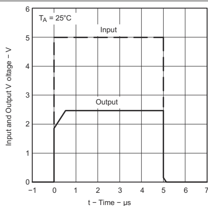
图 6-9. 脉冲响应
