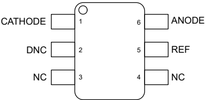
图 5-3. DRL 封装、 6 引脚 SOT-563、TLA431 ( 顶视图 )
