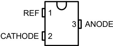
图 5-2. DBZ 封装、 3 引脚 SOT-23、TLA432 ( 顶视图 )
