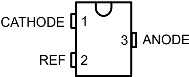
图 5-1. DBZ 封装、 3 引脚 SOT-23、TLA431 ( 顶视图 )
