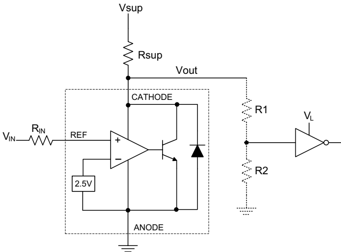
图 9-3. 比较器应用原理图
