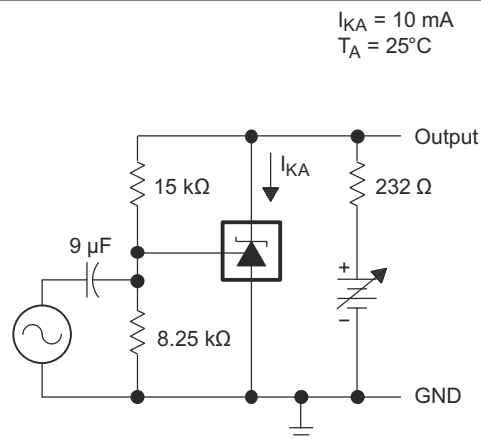
图 6-6. 电压放大测试电路
