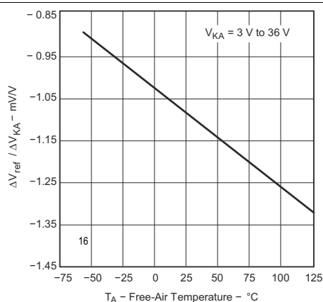
图 6-4. \Delta 基准电压与 \Delta 阴极电压之比与自然通风条件下的温度之间的关系
