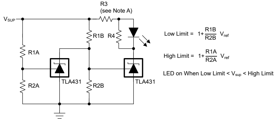
图 9-8. 电压监控器
