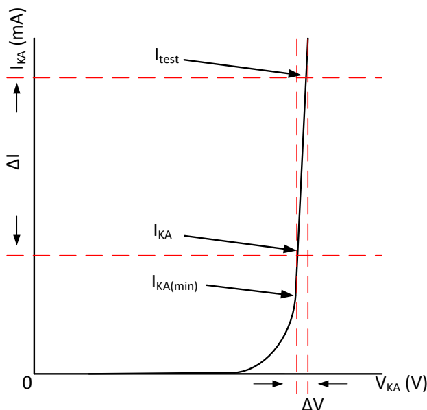
图 7-5. 动态阻抗
