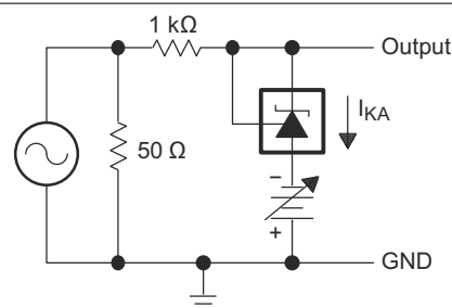
图 6-8. 基准阻抗测试电路
