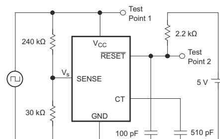
图 6-8. V_{CC} vs Output Test Circuit 1
