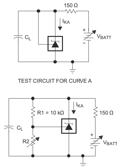
图 6-17. 稳定性边界条件测试电路
