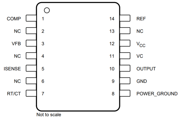
D 封装 14 引脚 SOIC 顶视图
