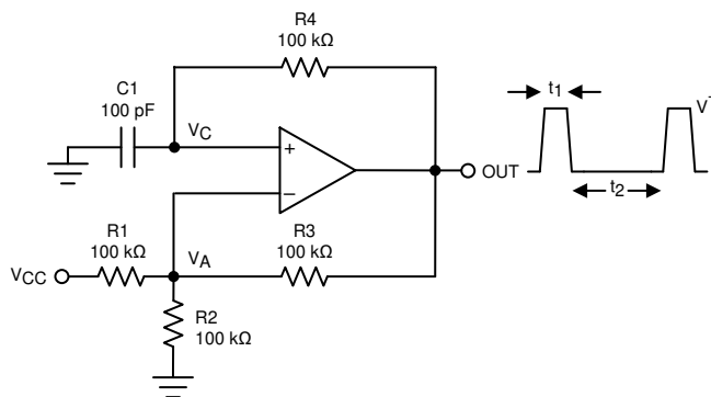
图 7-9. 方波振荡器
