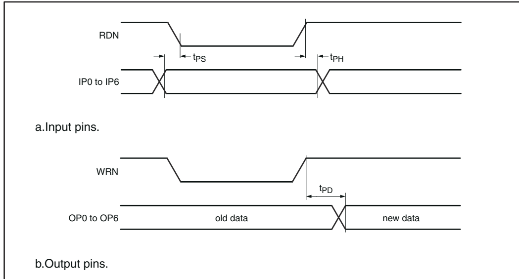
图 4-7. Port Timing
