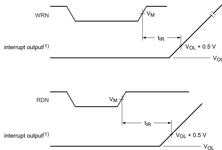
图 4-7. Port Timing
