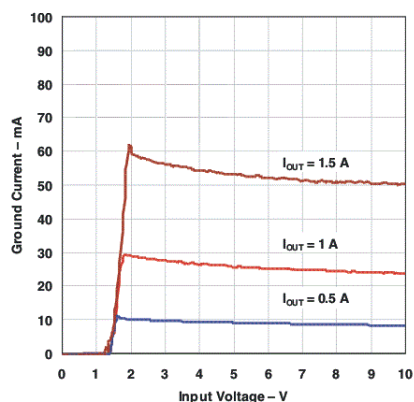
图 5-15. TL1963A 接地电流与输入电压间的关系 (旧芯片)
