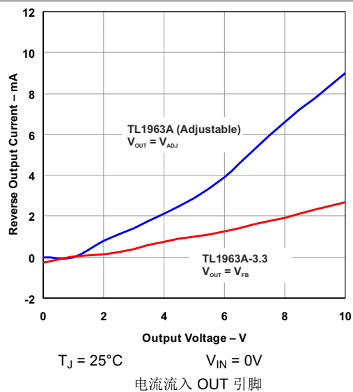
图 5-30. 反向输出电流与输出电压间的关系 (旧芯片)
