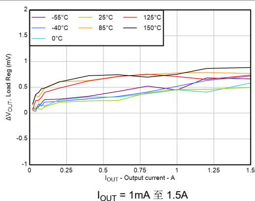
图 5-36. 负载调整率与温度间的关系 (新芯片)
