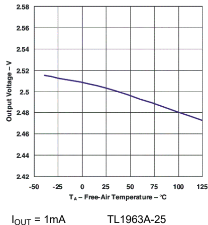
图 5-8. TL1963A-25 输出电压与温度间的关系 (旧芯片)
