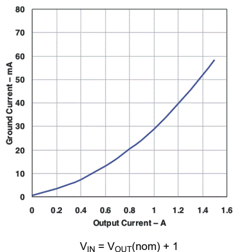
图 5-20. 接地电流与输出电流间的关系 (旧芯片)
