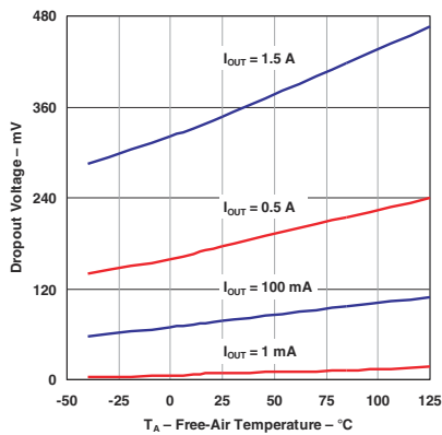
图 5-3. 压降电压与温度之间的关系 ( 旧芯片 )
