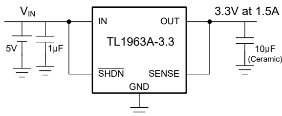
图 7-2. 4.3V 至 3.3V 稳压器
