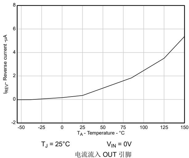
图 5-31. 反向输出电流与温度间的关系 (新芯片)
