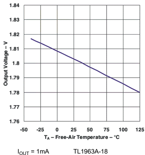
图 5-7. TL1963A-18 输出电压与温度间的关系 (旧芯片)
