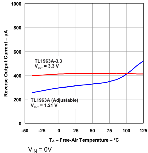
图 5-32. 反向输出电流与温度间的关系 (旧芯片)
