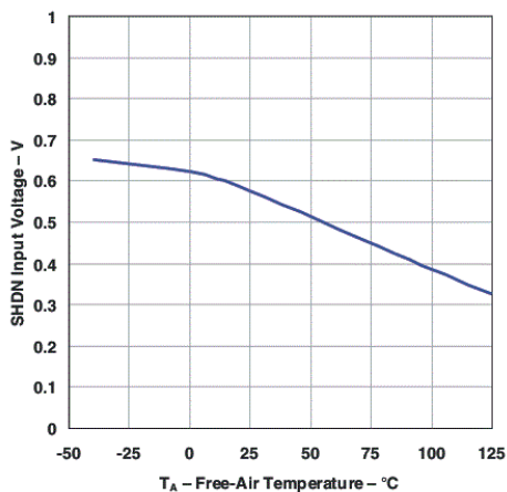
图 5-25. \overline{\text{SHDN}} 阈值 (导通至关断) 与温度间的关系 (旧芯片)
