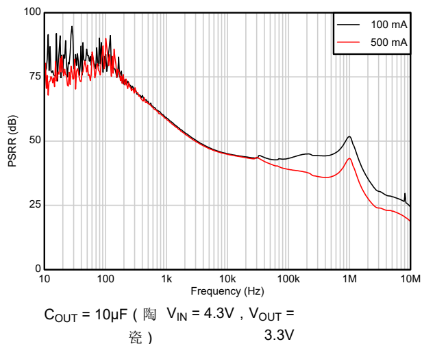
图 5-34. 纹波抑制与频率间的关系 (新芯片)
