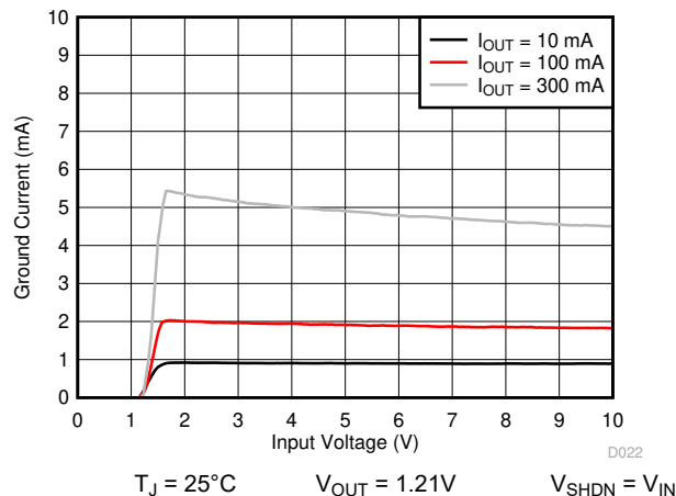
图 5-14. TL1963A 接地电流与输入电压间的关系 (旧芯片)
