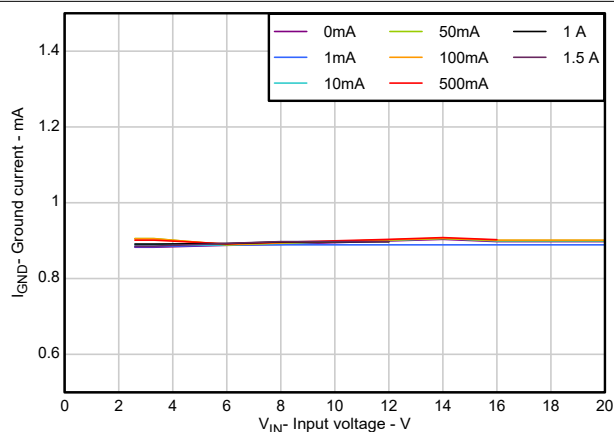
图 5-16. TL1963A-33 接地电流与输入电压间的关系 (旧芯片)
