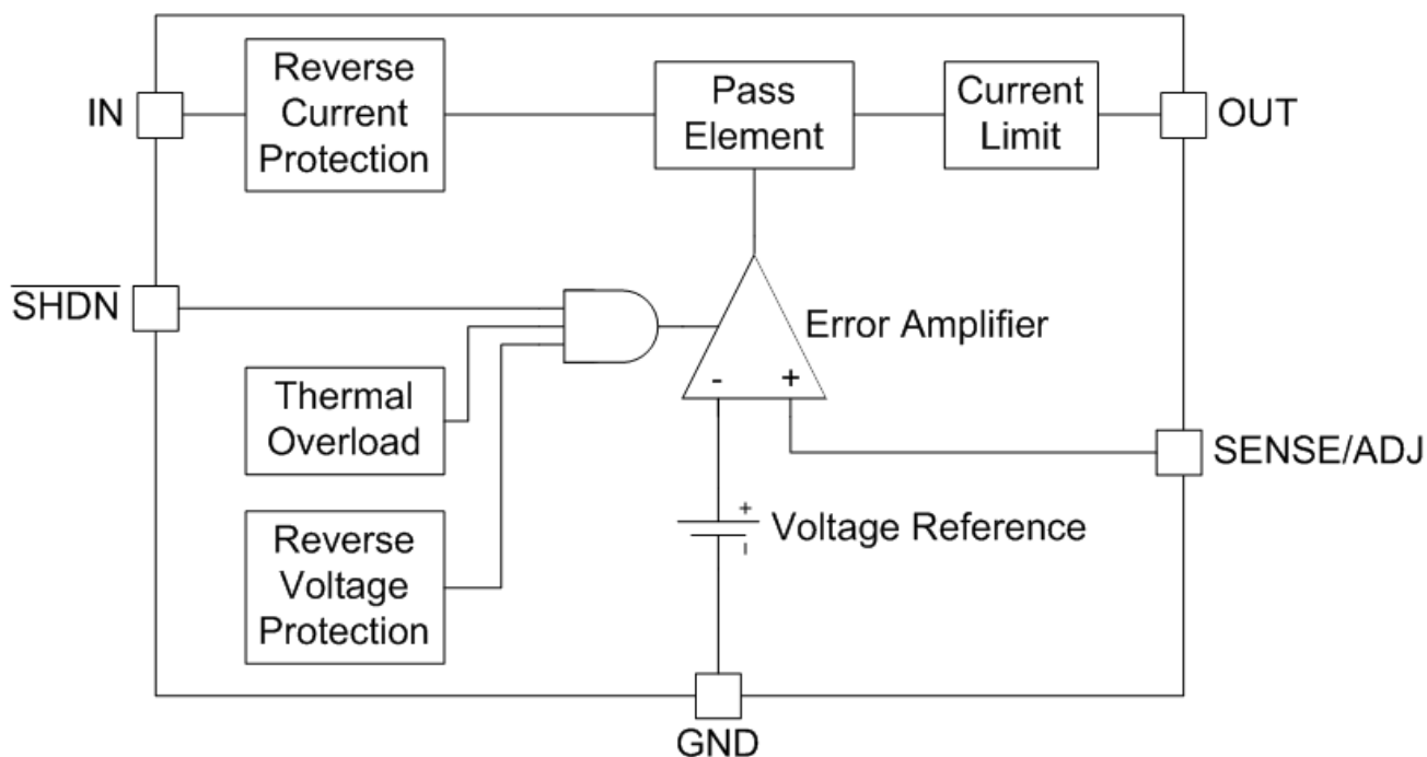
图 6-1. 功能方框图
