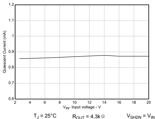
图 5-13. 静态电流与输入电压之间的关系 (新芯片)
