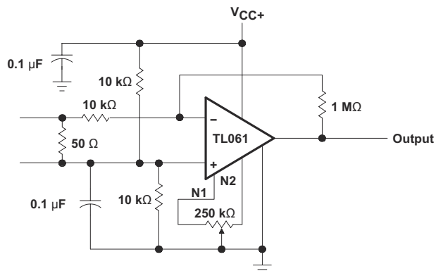
图 9-8. AC Amplifier
