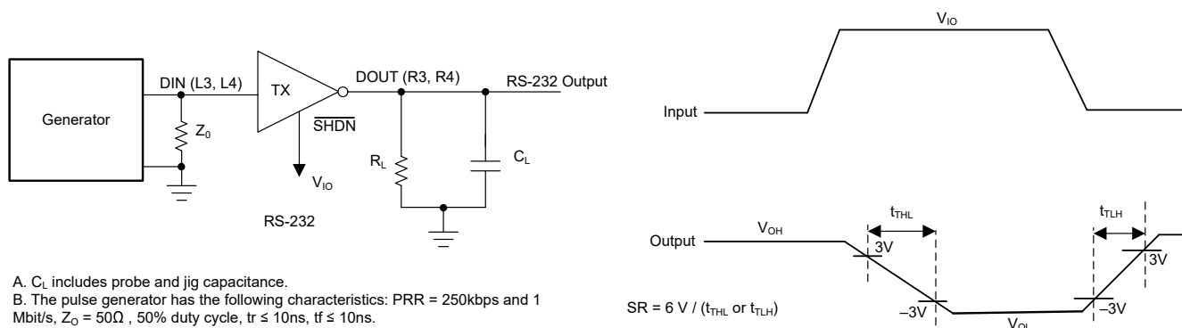
图 6-16. RS-232 驱动器压摆率
