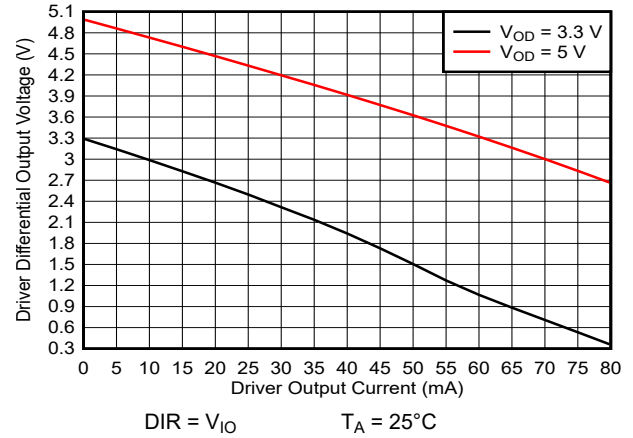
图 5-6. RS-485 驱动器差分输出电压与驱动器输出电流之间的关系
