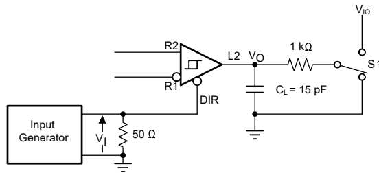
图 6-7. 半双工模式下 RS-485 接收器启用/禁用时间测量
