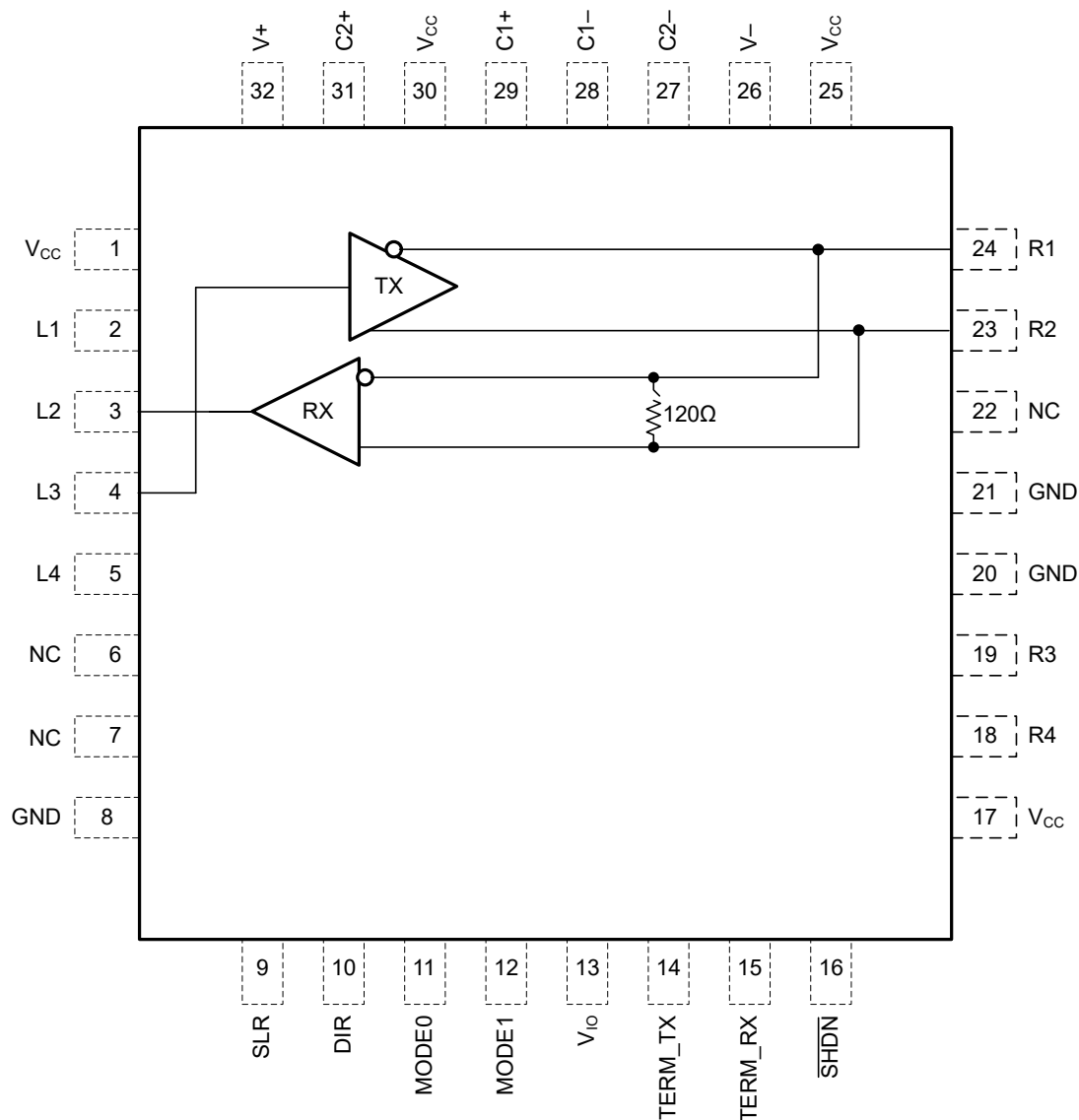
图 7-4. RS-485 半双工模式
