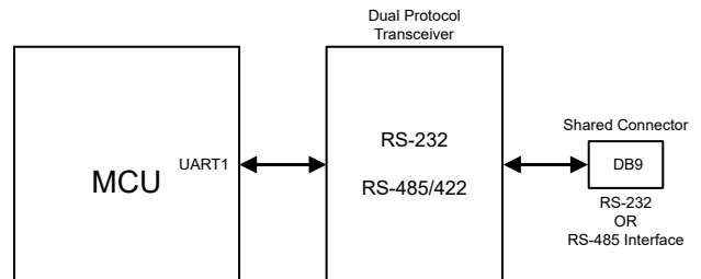
THVD4421 简化原理图
