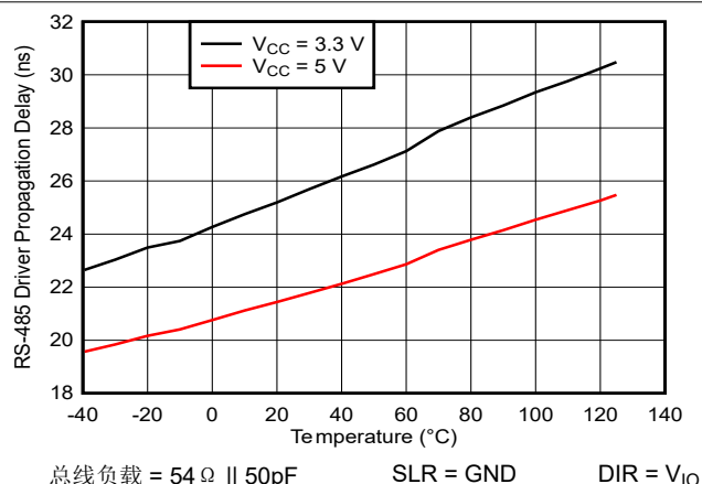
图 5-12. RS-485 20Mbps 驱动器传播延迟与温度间的关系
