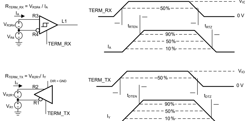
图 6-10. 端接电阻器开关测量
