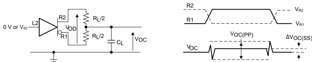
图 6-2. 具有 RS-485 负载的 RS-485 驱动器差分输出和共模输出测量
