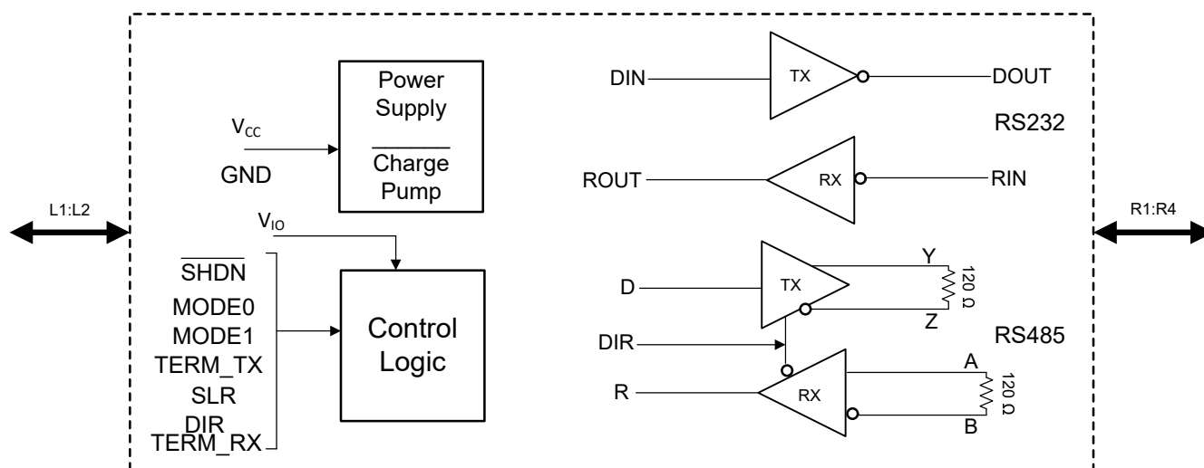
图 7-1. THVD4411 方框图
