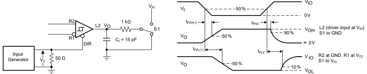
图 6-7. 半双工模式下 RS-485 接收器启用和禁用时间测量
