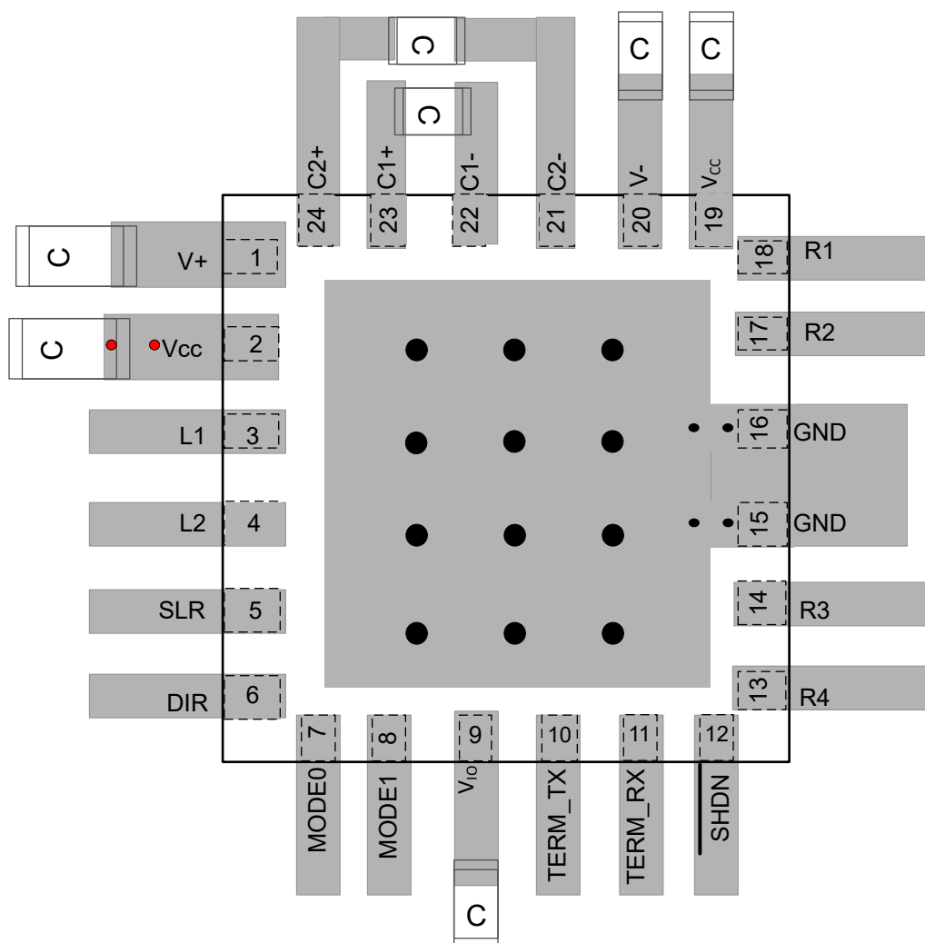
图 8-11. 布局示例
