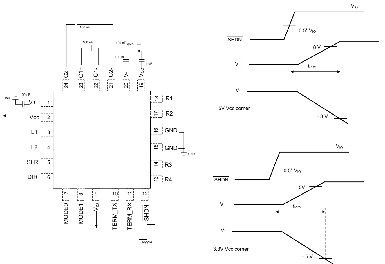
图 6-11. 从关断到 RS-232 就绪的时间
