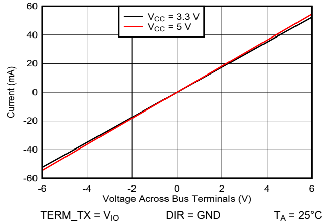
图 5-4. 端接开启时 R2-R1 总线引脚上的电压与电流之间的关系
