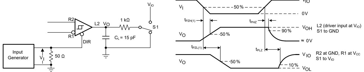
图 6-6. RS-485 接收器输出上升和下降时间以及传播延迟测量
