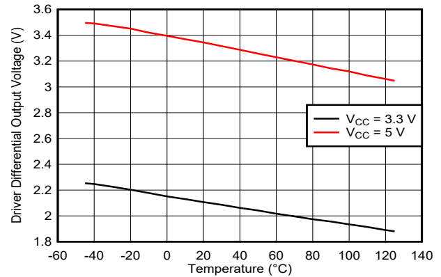
图 5-8. RS-485 驱动器差分输出电压与温度间的关系
