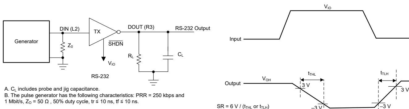
图 6-15. RS-232 驱动器压摆率
