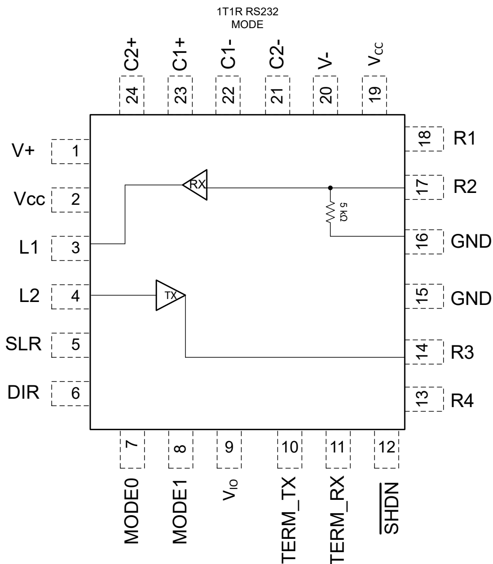
图 7-2. RS-232 模式
