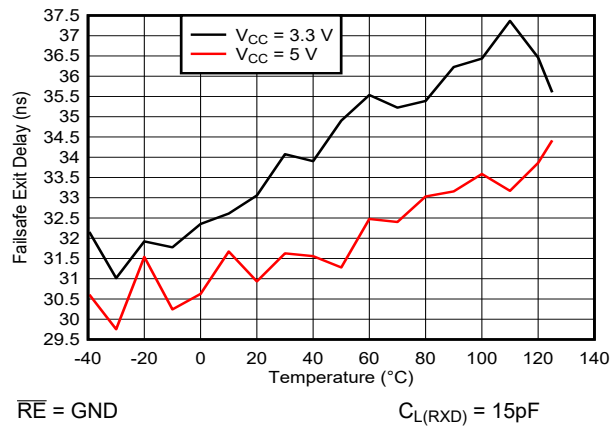
图 5-11. 失效防护退出延迟与温度间的关系
