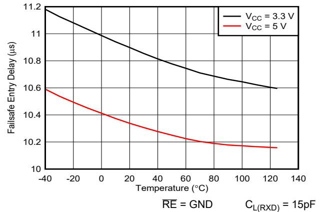
图 5-10. 失效防护进入延迟与温度间的关系
