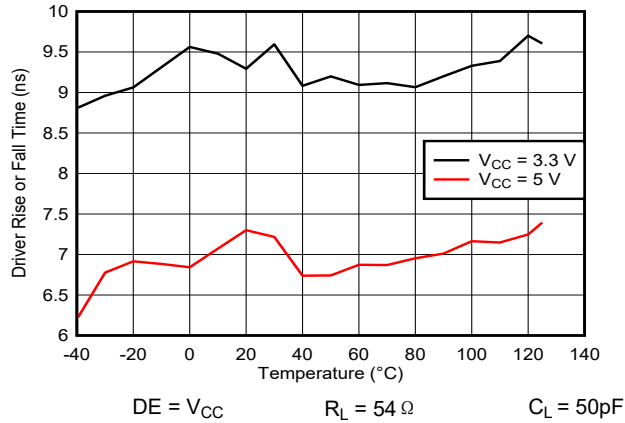
图 5-7. THVD2442 20Mbps 驱动器上升时间或下降时间与温度间的关系
