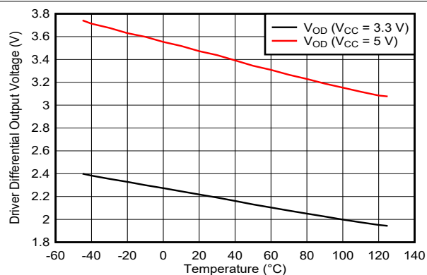
图 5-4. 驱动器差分输出电压与温度间的关系
