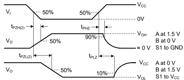
图 6-8. 驱动器被禁用情况下接收器启用次数的测量
