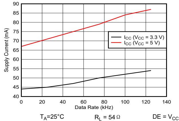
图 5-9. THVD2412 电源电流与信号速率间的关系
