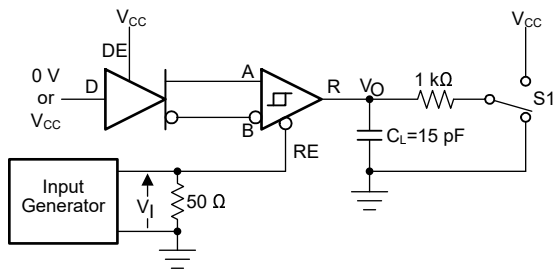
图 6-7. 驱动器已启用情况下接收器启用/禁用次数的测量
