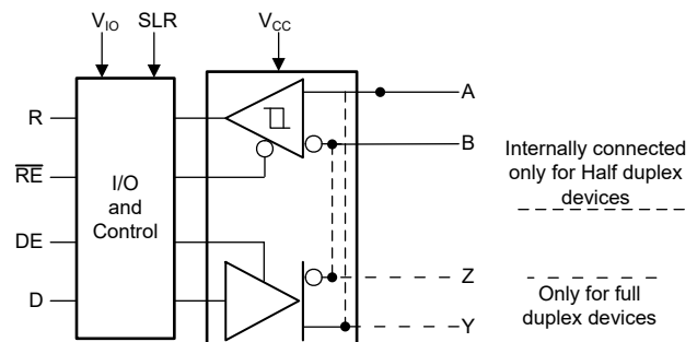
简化原理图
