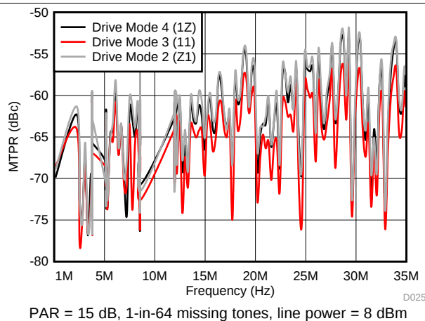
图 21. MTPR VDSL2-35b Profile
