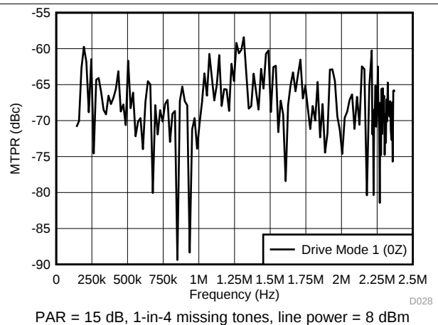
图 24. MTPR ADSL2+ Profile
