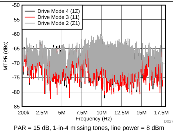
图 23. MTPR VDSL2-17a Profile
