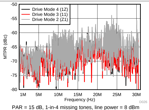
图 22. MTPR VDSL2-30a Profile
