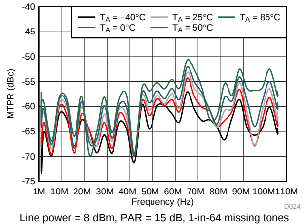
图 20. MTPR Over Temperature G.Fast 106-MHz Profile (Bias 01)
