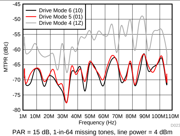
图 19. MTPR G.Fast 106-MHz Profile
