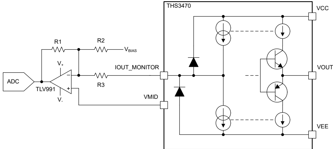
图 6-6. I_{OUT\_2048} 跨阻原理图
