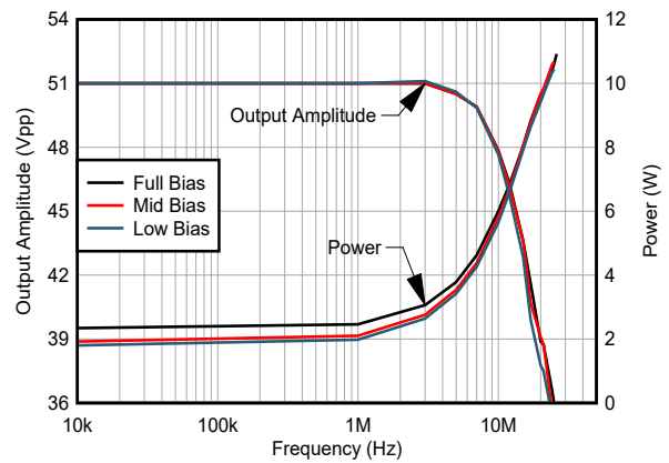
图 6-12. 大信号带宽与频率间的关系 ( R_F = 2k\Omega , R_S = 5\Omega , C_L = 1nF )
