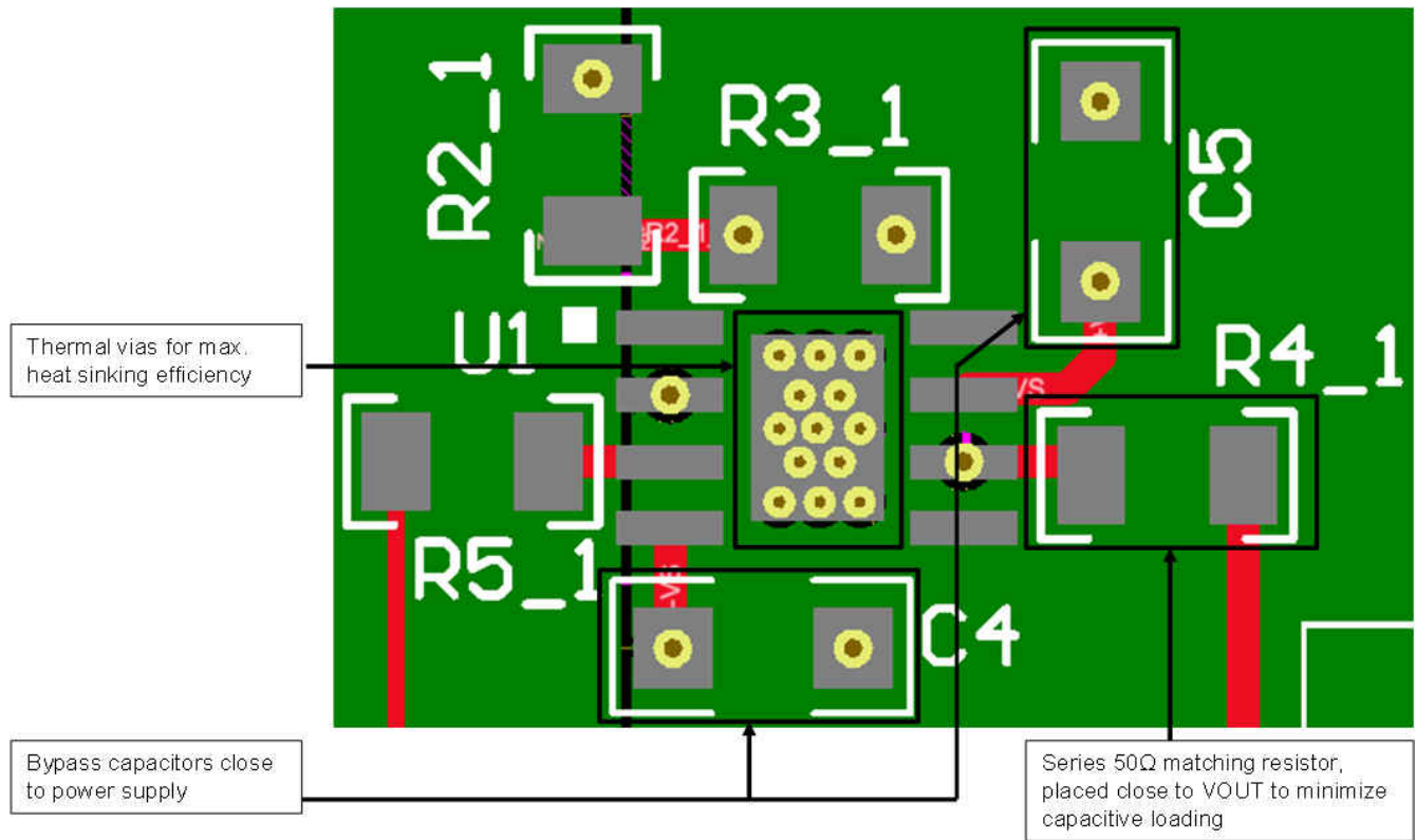
图 9-8. Layout Recommendation
